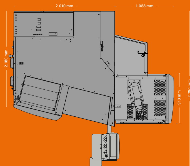
////// DIMENSIONI MACCHINA VGrind 360S con HPR 250
