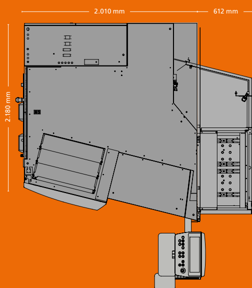
////// DIMENSIONI MACCHINA VGrind 360S con HP 170 o HC 4
