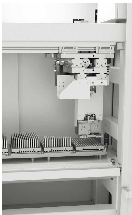
//////// DEPOSITO PALLET HP 170 per immagazzinare rapidamente fino a 900 utensili
