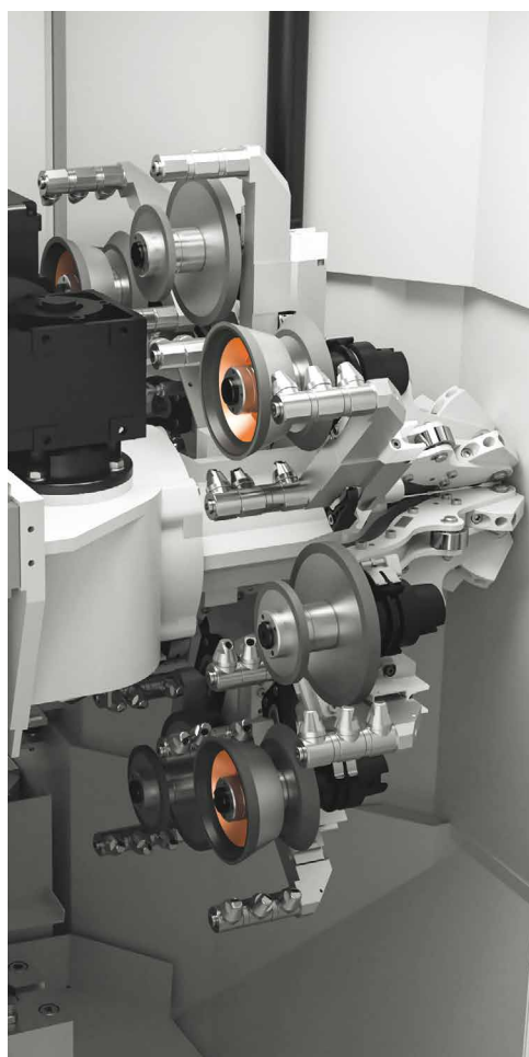
//////// DISPOSITIVO 8X PER CAMBIO MOLE DI AFFILATURA con ugelli per il refrigerante
