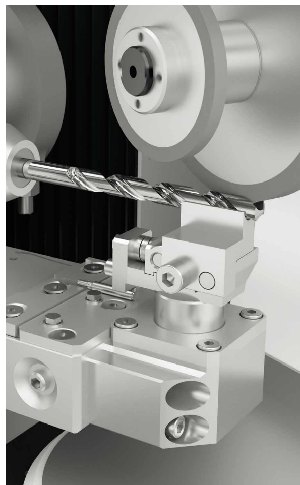
///// La lunetta, dotata di corsa automatica, assicura un risultato di affilatura ottimale in caso di utensili più lunghi
